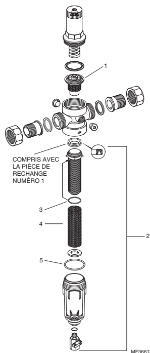
Fig. 5. Schéma des pièces de rechange.
