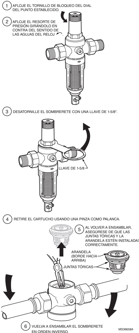
Fig. 4. Remplazar el cartucho FK06.
