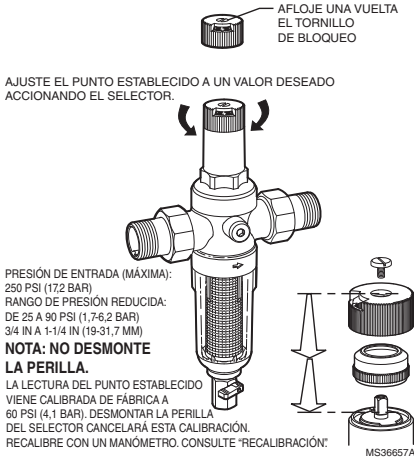
Fig. 2. Cambiar presión de salida.
