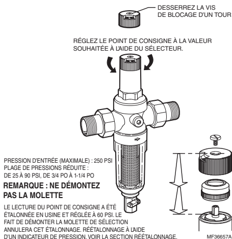
Fig. 2. Modification de la pression de sortie.
