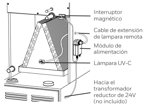
Fig. 6. Fije el módulo de alimentación a la unidad de tratamiento de aire o al conducto con tornillos largos. No los apriete en exceso.
