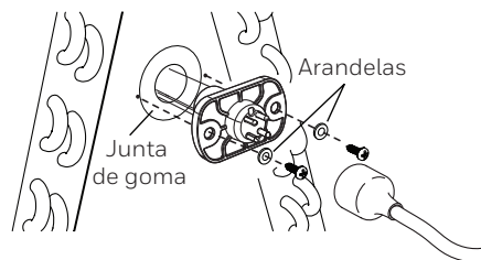
Fig. 5. Inserte la lámpara en el orificio ciego de la placa delta y fíjela con tornillos y arandelas. Conecte el cable de extensión de la lámpara remota.
