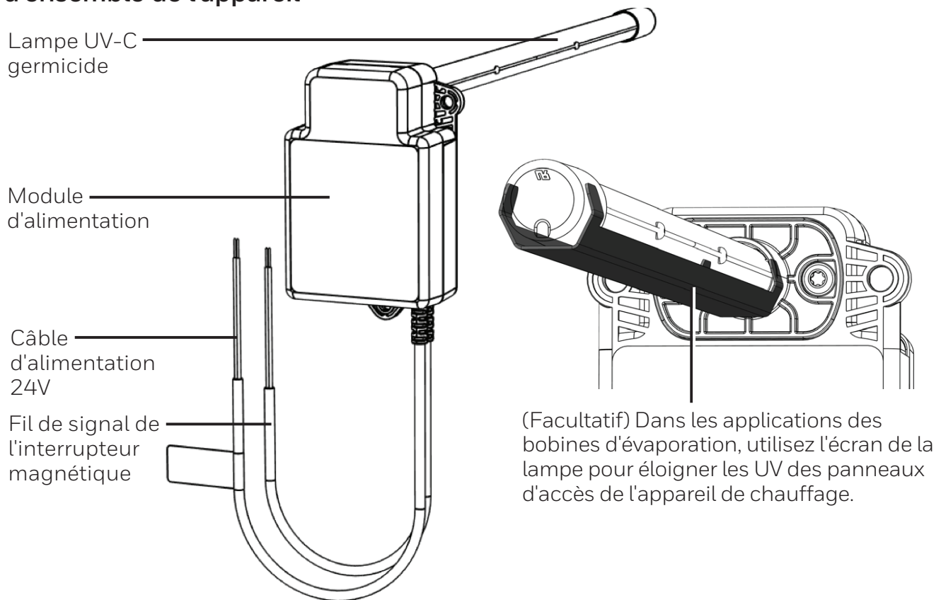
Fig. 1. Identification des composants de l'appareil.
