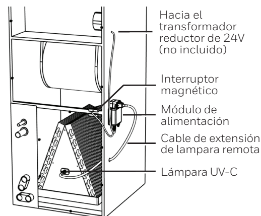
Fig. 4. Instalación de la unidad de tratamiento de aire.
