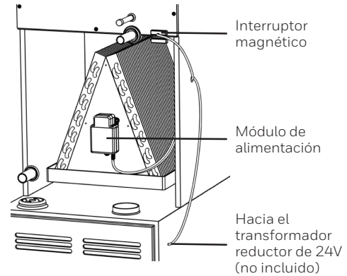
Fig. 9. Conecte el interruptor magnético y el cable de alimentación.
