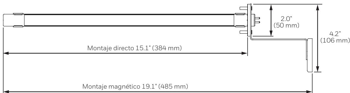
Fig. 2. Espacios mínimos.
