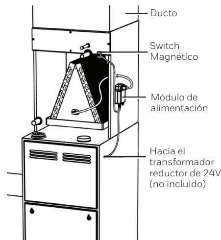
Fig. 3. Instalación de la calefacción/serpentín con carcasa.
